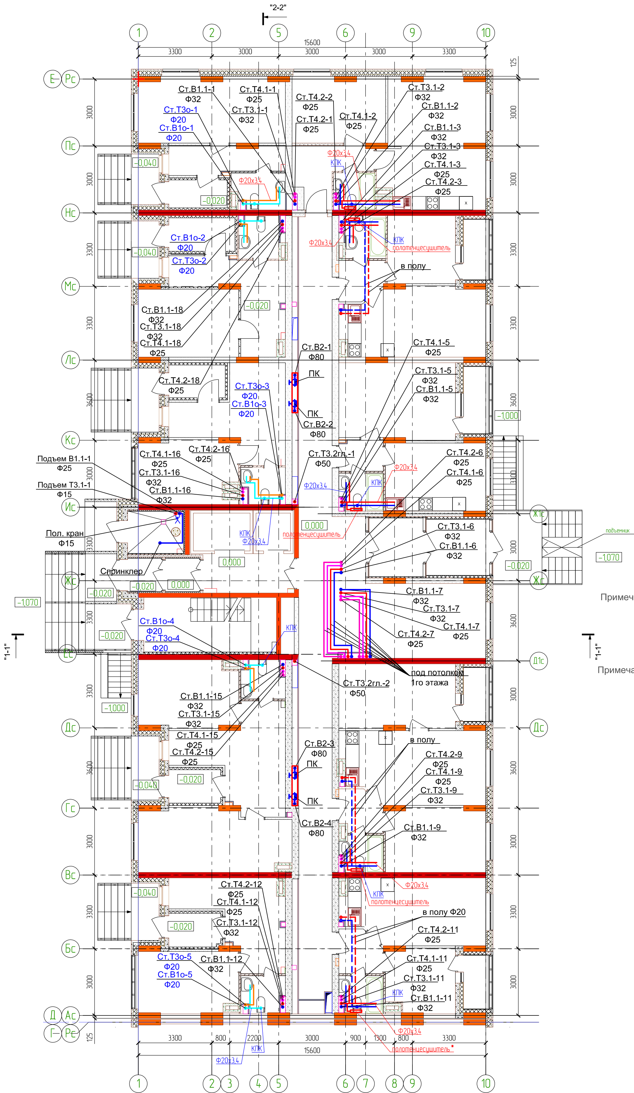
План 1 этажа секции в осях 1-10 и Д-Е с сетями В1.1, В2, В1о, Т3.1, Т3.2, Т3о, Т4.1, Т4.2
